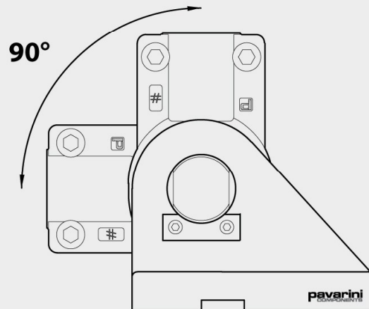
ACCOPPIAMENTO IKB CON TAPR...CE ASSEMBLING IKB WITH TAPR...CE
