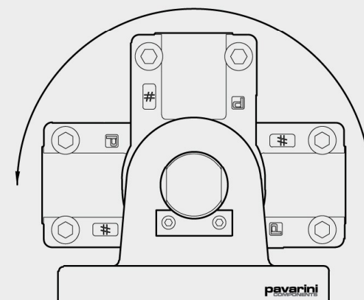
ACCOPPIAMENTO IKA CON TAPR...CE ASSEMBLING IKA WITH TAPR...CE
